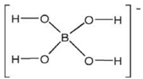
BORAX
